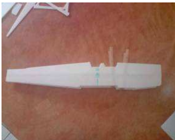
Collage de l'âme centrale dépron 6 mm
